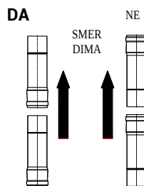
Slika 7. Način montaže dimnih cevi
